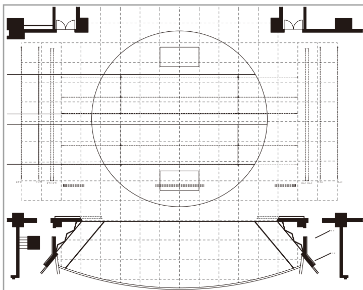
舞台平面図
