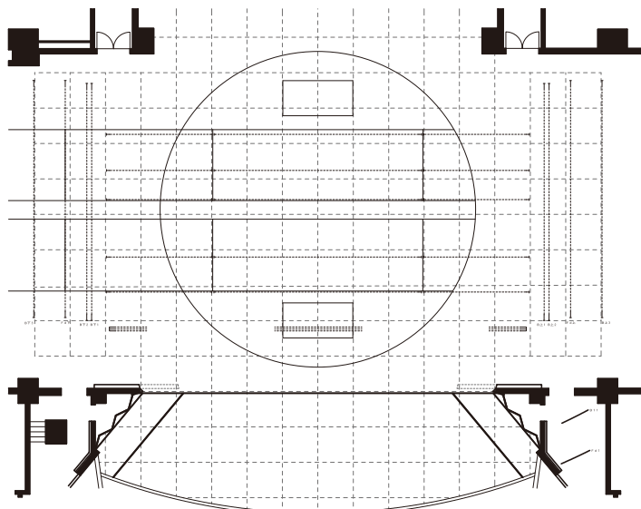
舞台平面図
